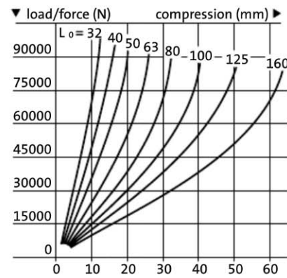
2461.4.125. Ø 125/70 Shore A
